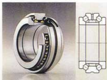
Aksial-vinkelkontaktkugleleje dobbeltvirkende
