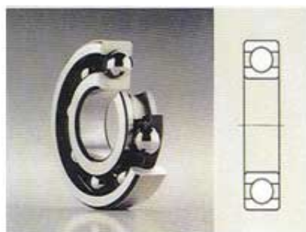
Sporkugleleje enradet
