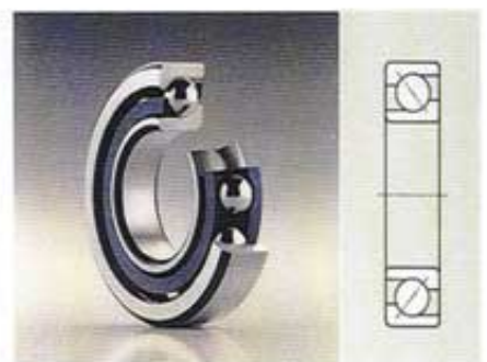
Vinkelkontaktkugleleje enradet
