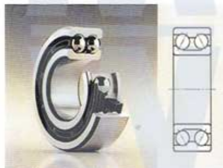
Vinkelkontaktkugleleje toradet
