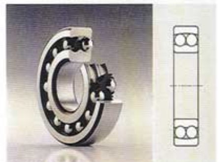
Sfærisk kugleleje
